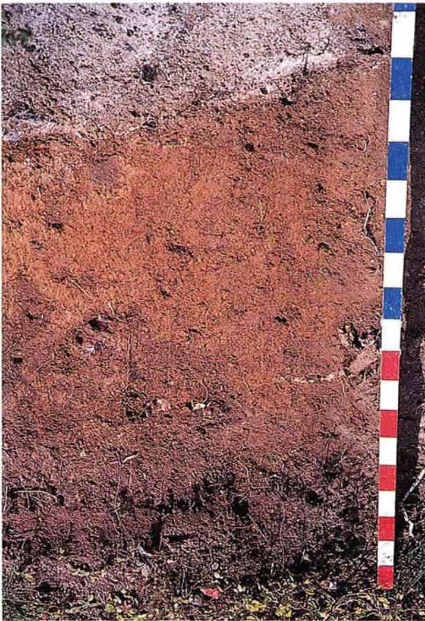
13 Braunerde aus Vulkantuff (Bausenberg, Osteifel).
